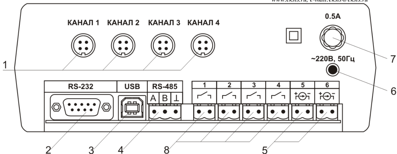
Рисунок 3.3 Задняя панель приборов ИВГ-1 /1-С, ИВГ-1 /2-С.
